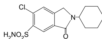
Clorexolone (Oxoisindoles)
