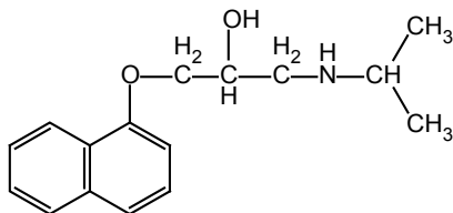
Propranolol
