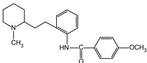
Encainide
