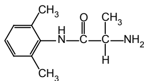
Tocainide
