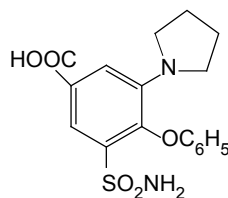
Piretanide
