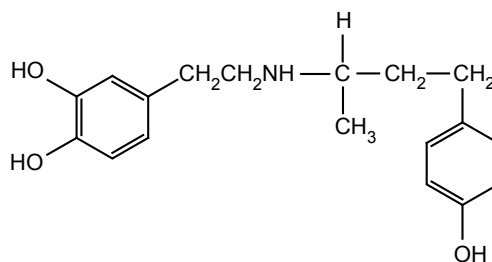
e. Dobutamine
