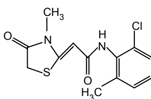
Ralitoline
