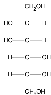
Mannitol
