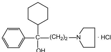
1-Cyclohexyl-1-phenyl-3-pyrrolidin-1-yl-1-propanol HCl
