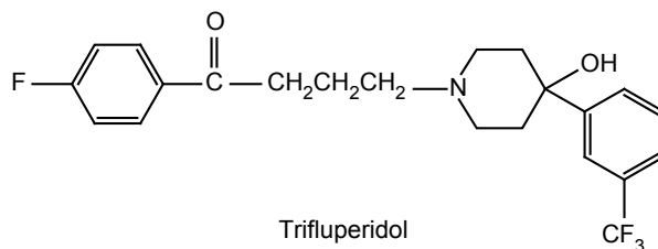
Haloperidol
