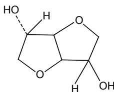
Isosorbide
